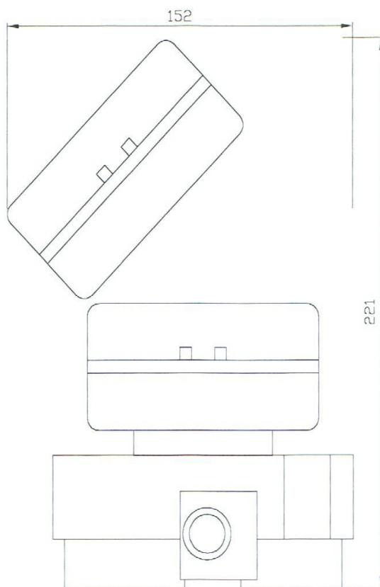
ULTRAFLOW monteret med regneværk
