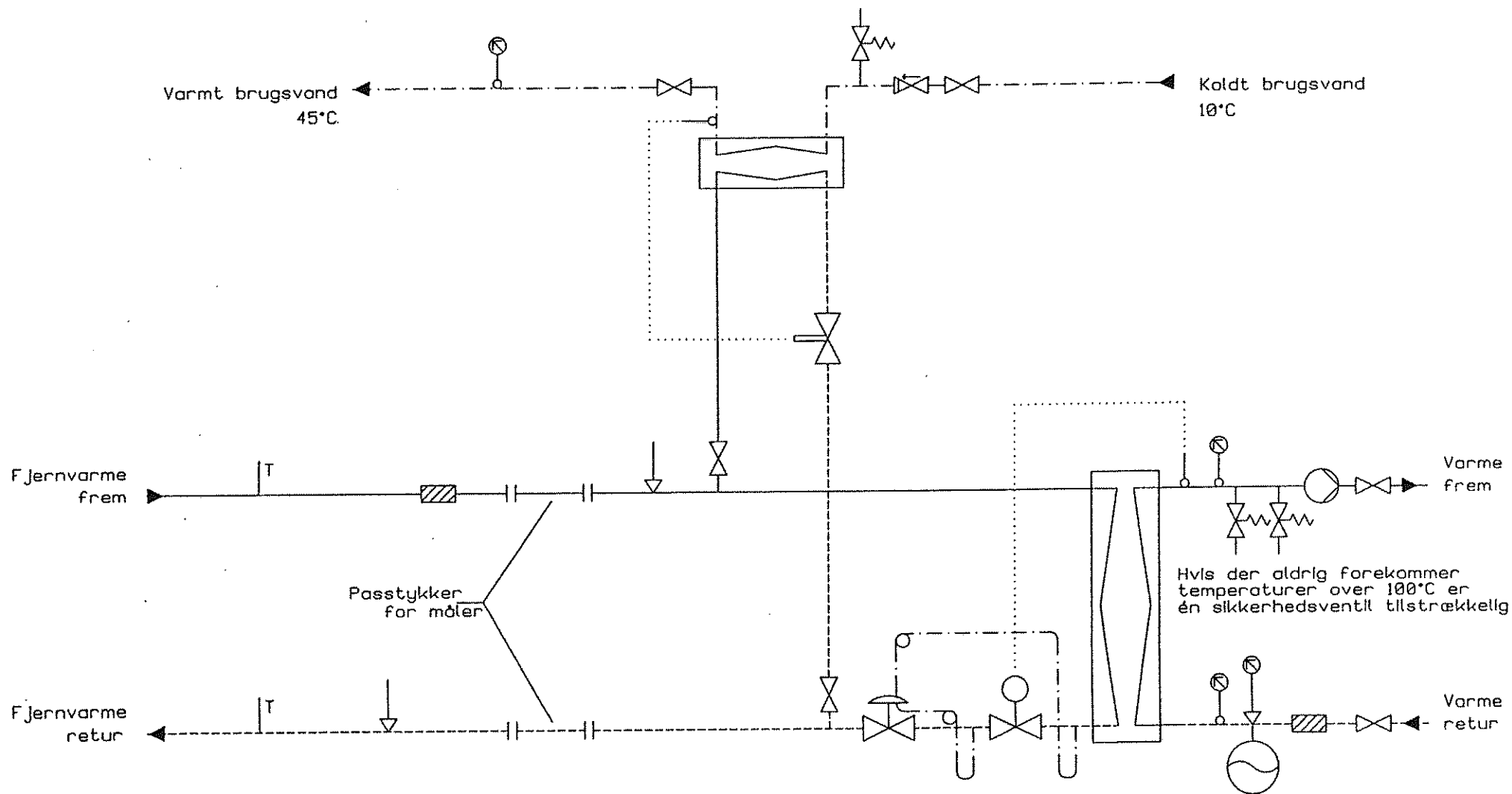
Varme anlæg med veksler og brugsvandsveksler.
